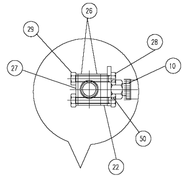
DETAIL-J
